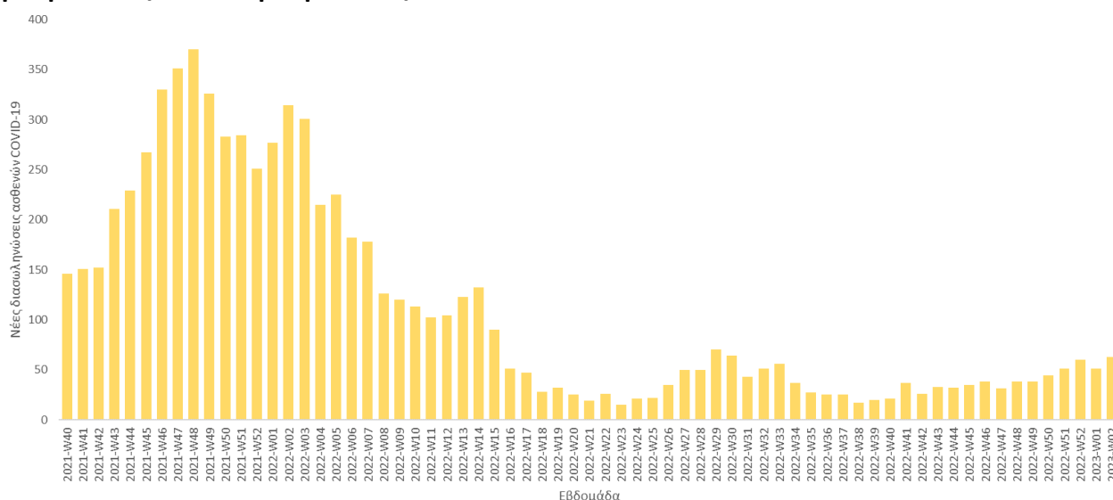
Διάγραμμα 9. Εβδομαδιαίος αριθμός νέων διασωληνώσεων ασθενών COVID-19, σύνολο χώρας, εβδομάδα 40/2021 – εβδομάδα 02/2023
