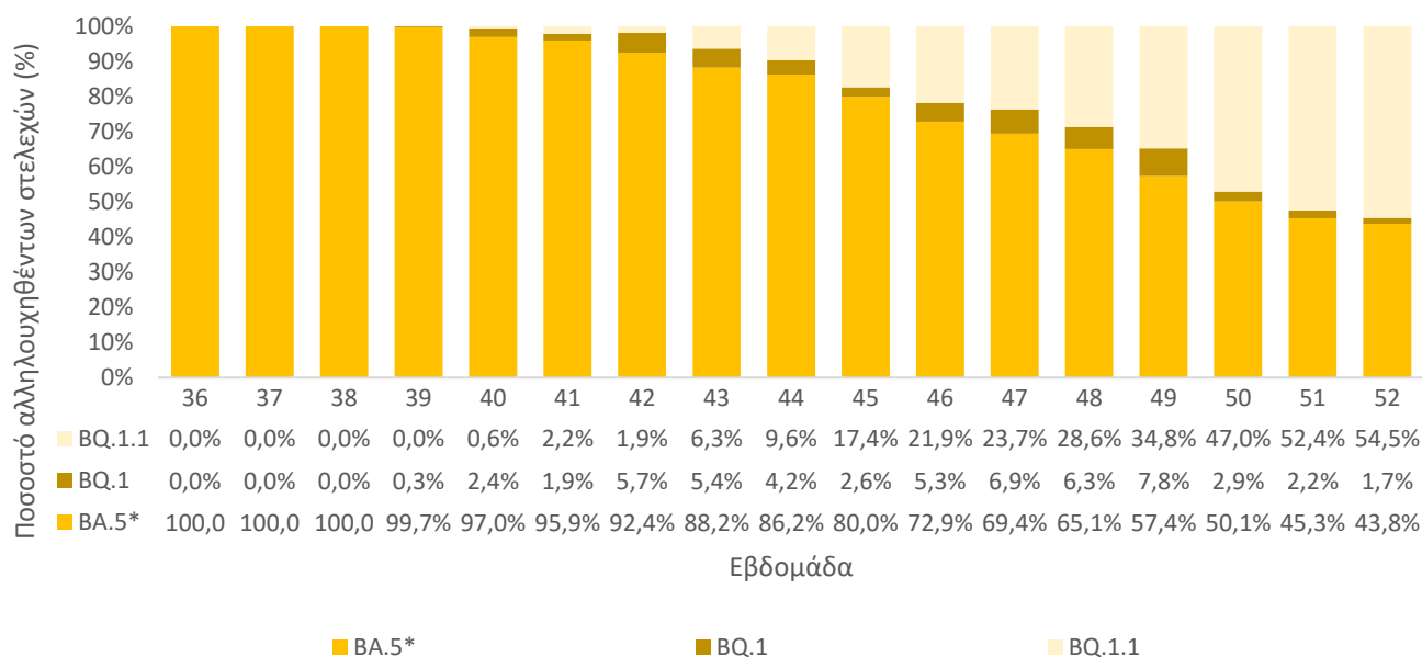
Διάγραμμα 17. Ποσοστό αλληλουχισθέντων δειγμάτων με απομονωθέν στέλεχος BA.5 ανά υπο-παραλλαγή επιδημιολογικού ενδιαφέροντος, ανά εβδομάδα, έως 01/01/2023
