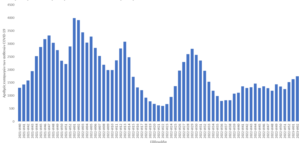
Διάγραμμα 8. Νέες εισαγωγές κρουσμάτων με λοίμωξη COVID-19 στα νοσοκομεία της επικράτειας ανά εβδομάδα, εβδομάδα 40/2021 – εβδομάδα 02/2023
