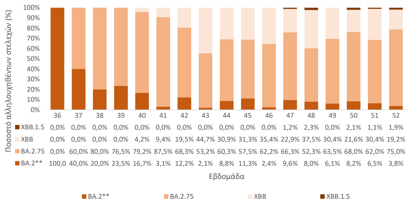
Διάγραμμα 18. Ποσοστό αλληλουχισθέντων δειγμάτων με απομονωθέν στέλεχος BA.2 ανά υπο-παραλλαγή επιδημιολογικού ενδιαφέροντος, ανά εβδομάδα, έως 01/01/2023
