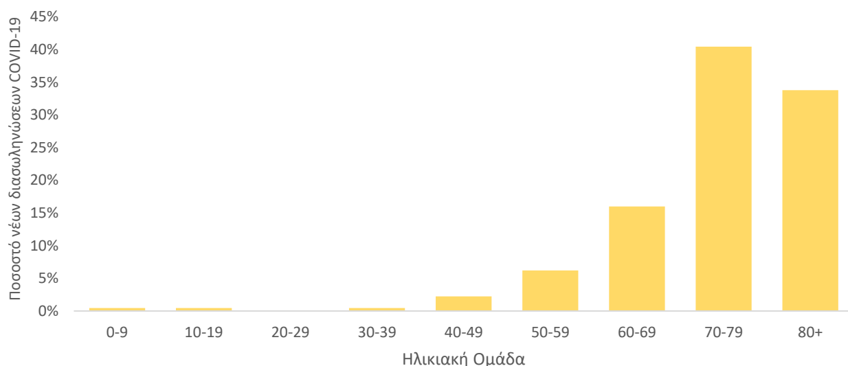
Διάγραμμα 10. Ποσοστό νέων διασωληνώσεων ασθενών με λοίμωξη COVID-19 στα νοσοκομεία της επικράτειας ανά ηλικιακή ομάδα, εβδομάδα 51/2022 – εβδομάδα 02/2023
